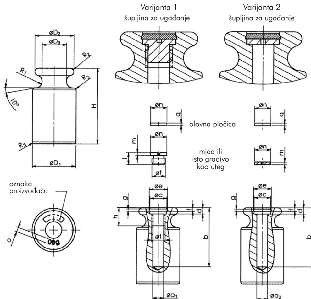
Slika A.1 Primjeri valjkastih utega
